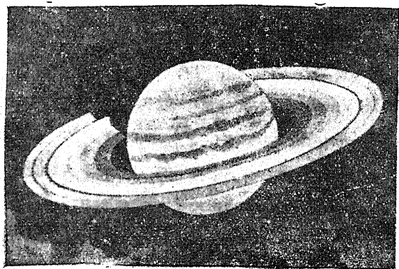
चित्र १—शनि का वलय
